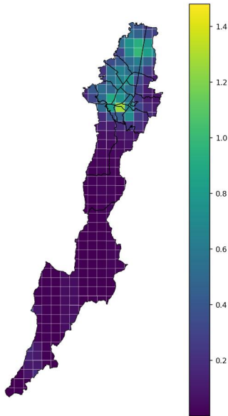
Proxy advectivo NO2 2023
