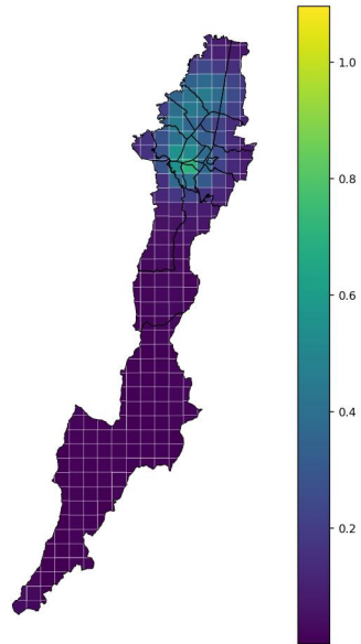
Proxy advectivo O3 2023
