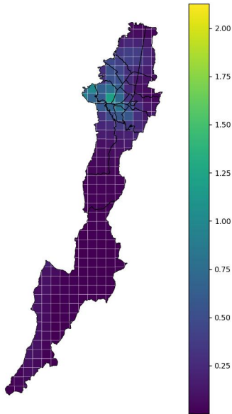
Proxy advectivo PM2.5 2023
