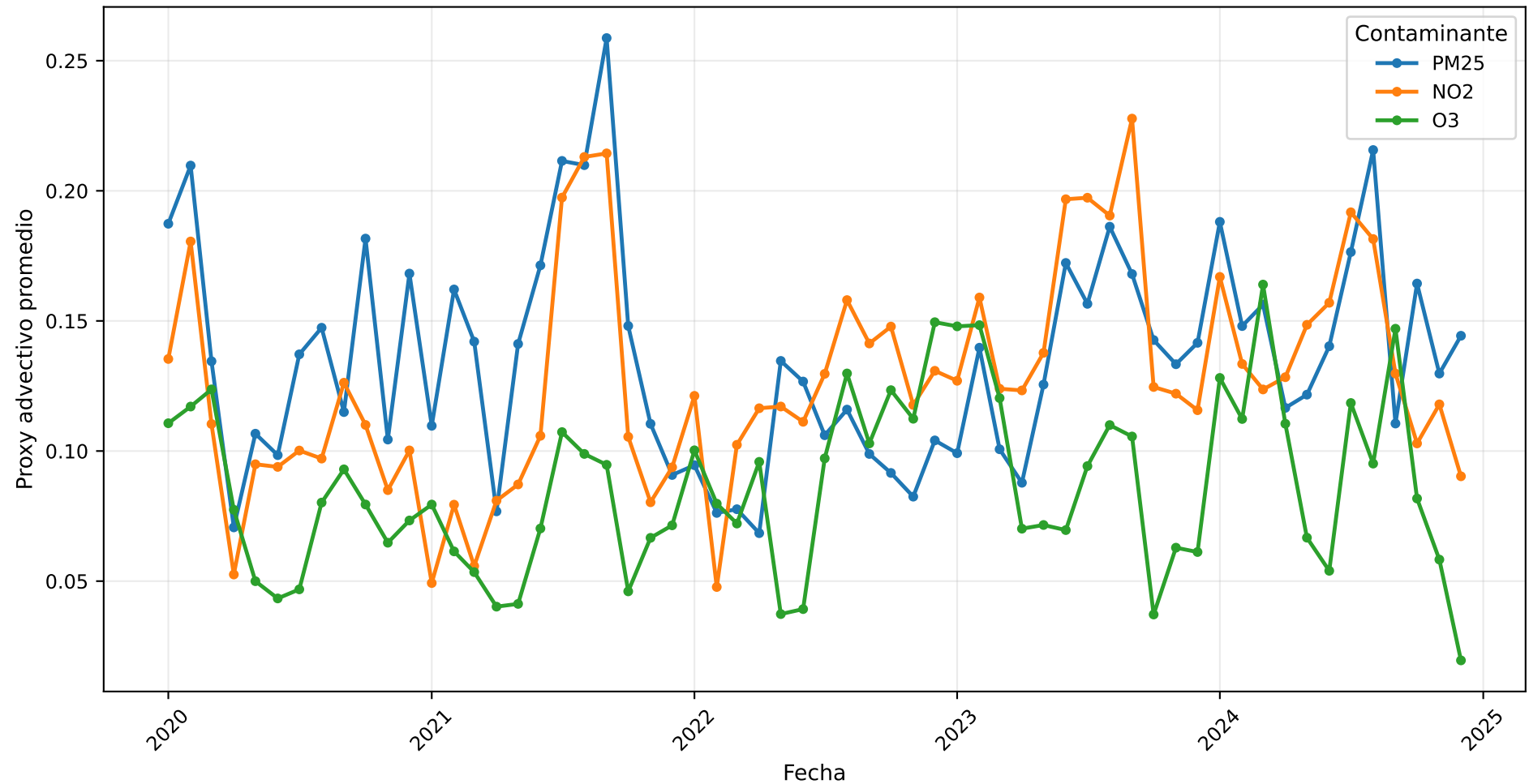
Promedio mensual del proxy advectivo por contaminante (escala por km)
