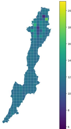
Superficie central O3 2021
