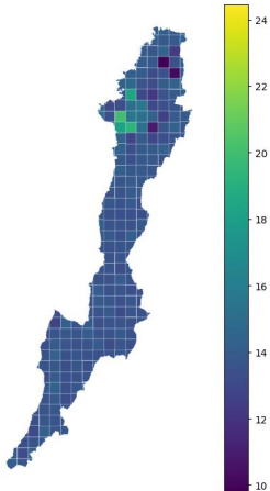
Superficie central PM2.5 2021
