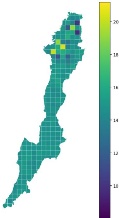
Superficie central NO2 2021
