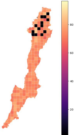
Incertidumbre PM2.5 2023
