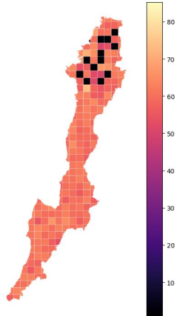
Incertidumbre O3 2023
