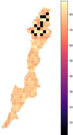
Incertidumbre NO2 2023
