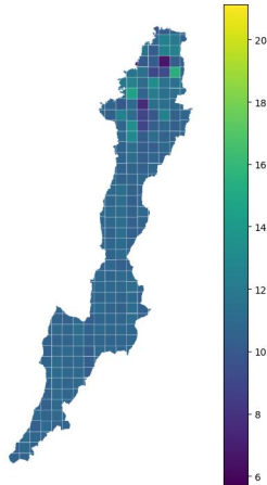
Superficie central O3 2022
