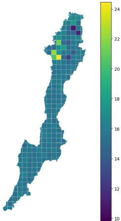
Superficie central PM2.5 2022
