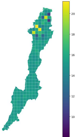
Superficie central NO2 2022
