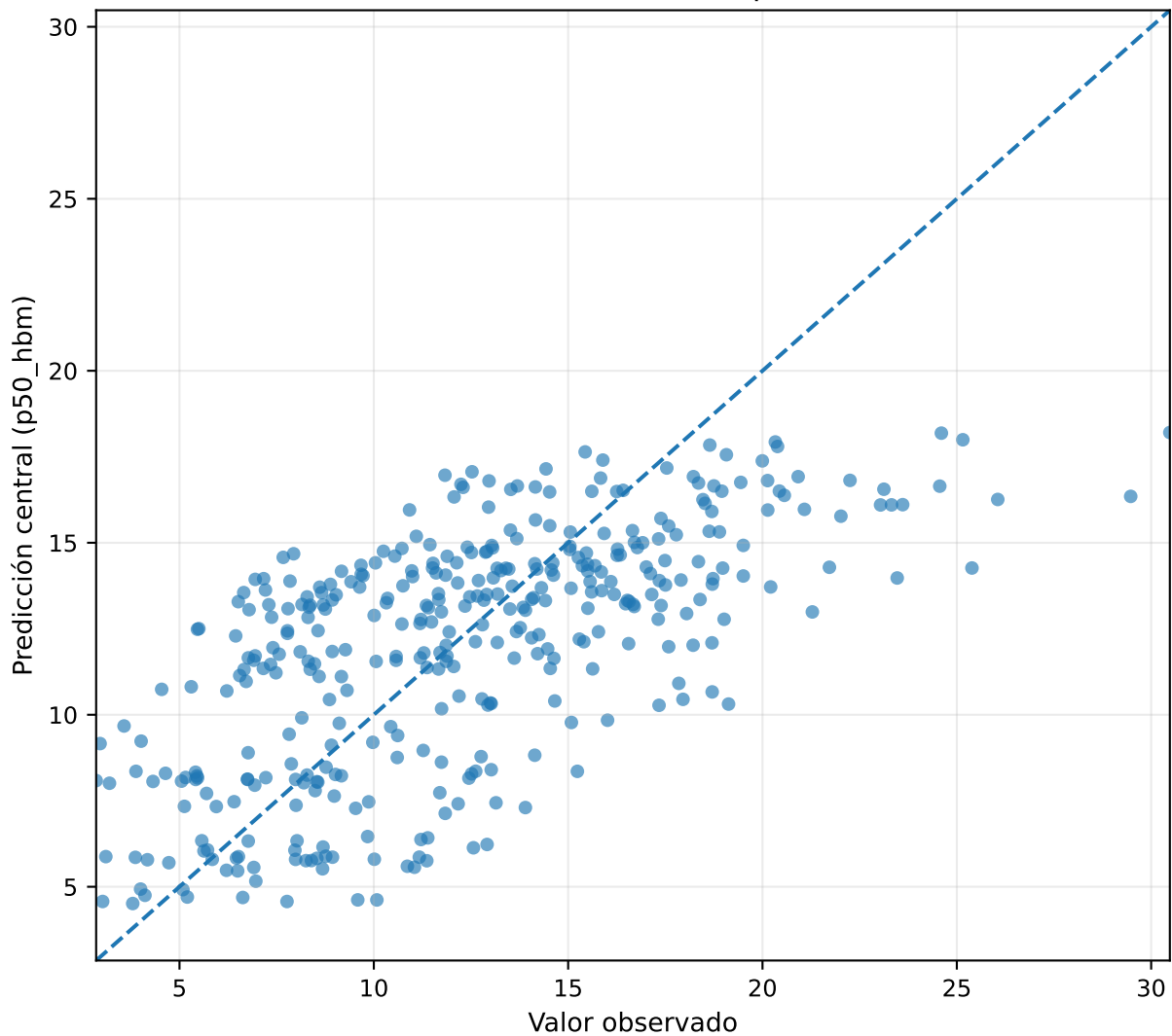
HBM O3: observado vs. predicho
