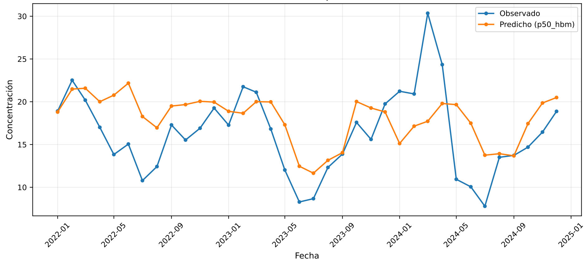
Serie mensual observada vs. predicha - HBM PM2.5
