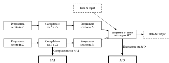
Figura 1.7: schema grafico soluzione ibrida
