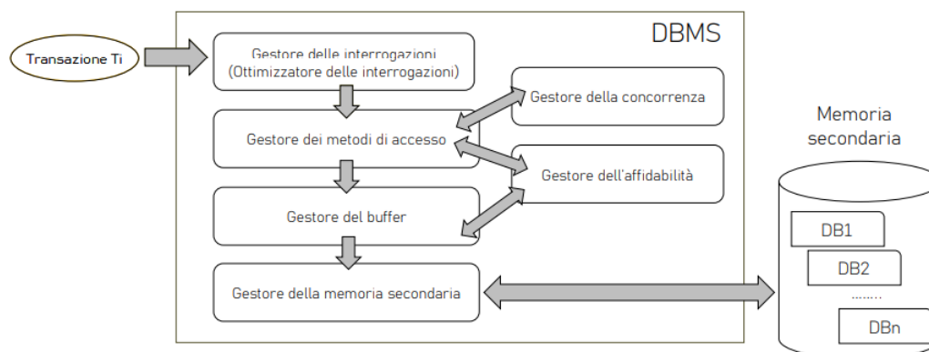
Figura 1.4: Architettura di riferimento di un DBMS.
