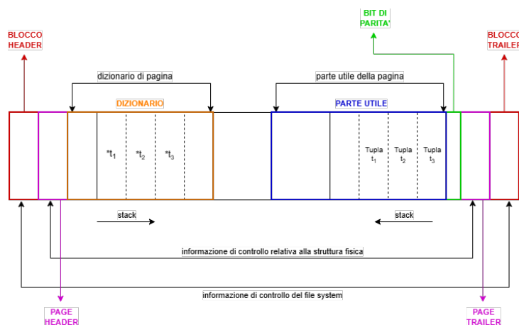
Figura 3.2: organizzazione di una pagina
