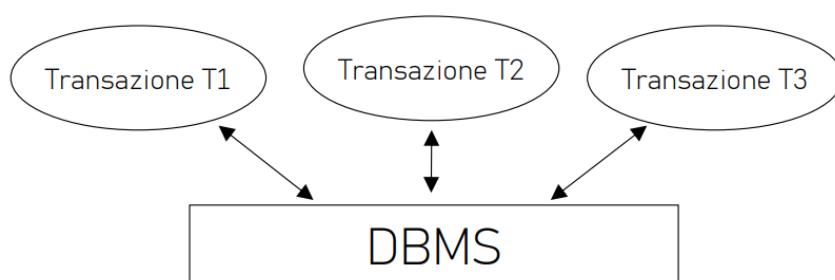
Figura 1.2: Ssistema transazionale
