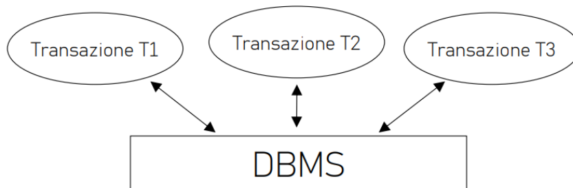
Figura 1.1: Sistema transazionale
