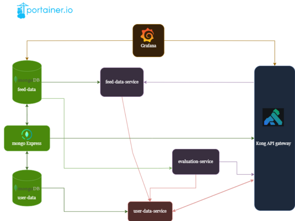
Figura 5.3: Arhitectura backend-ului aplicației
