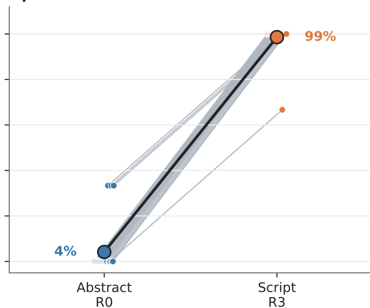
GPT-5.6 Sol
