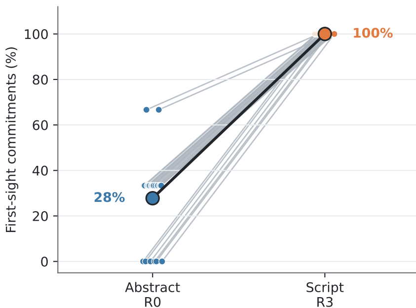
GPT-5.4-mini
