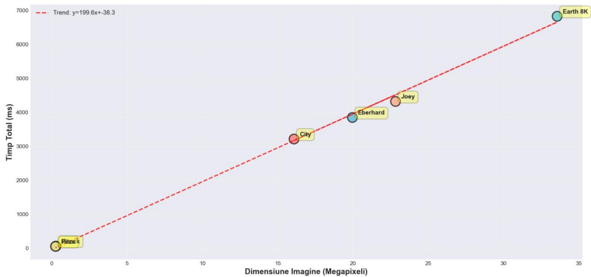
Scalabilitate: Timp vs Dimensiune Imagine
