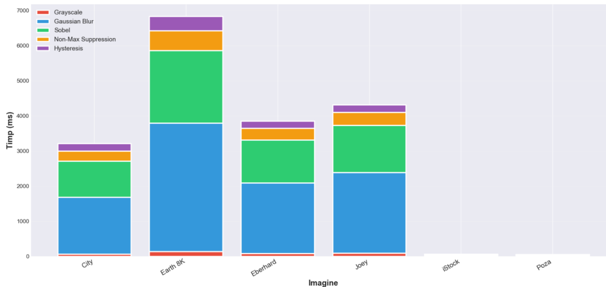
Scalabilitate: Timp vs Dimensiune Imagine
