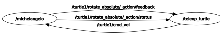
Figura 1: Gráfico de nodos y temas en ROS2 usando rqt_graph
