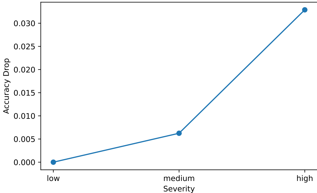
pamap2 CNN1D noise robustness
