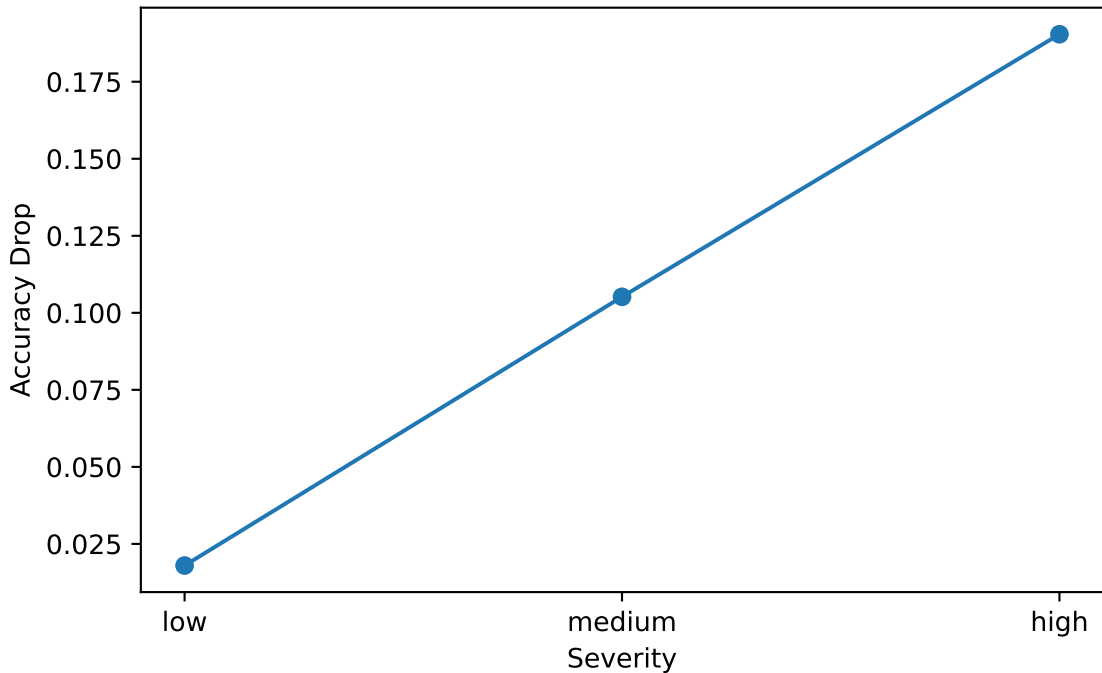
pamap2 Flatten_LSTM noise robustness
