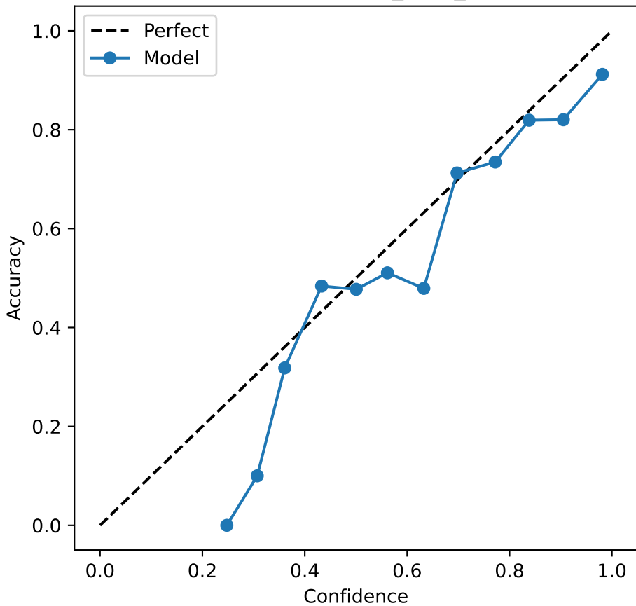
pamap2 Improved_GNN_LSTM
