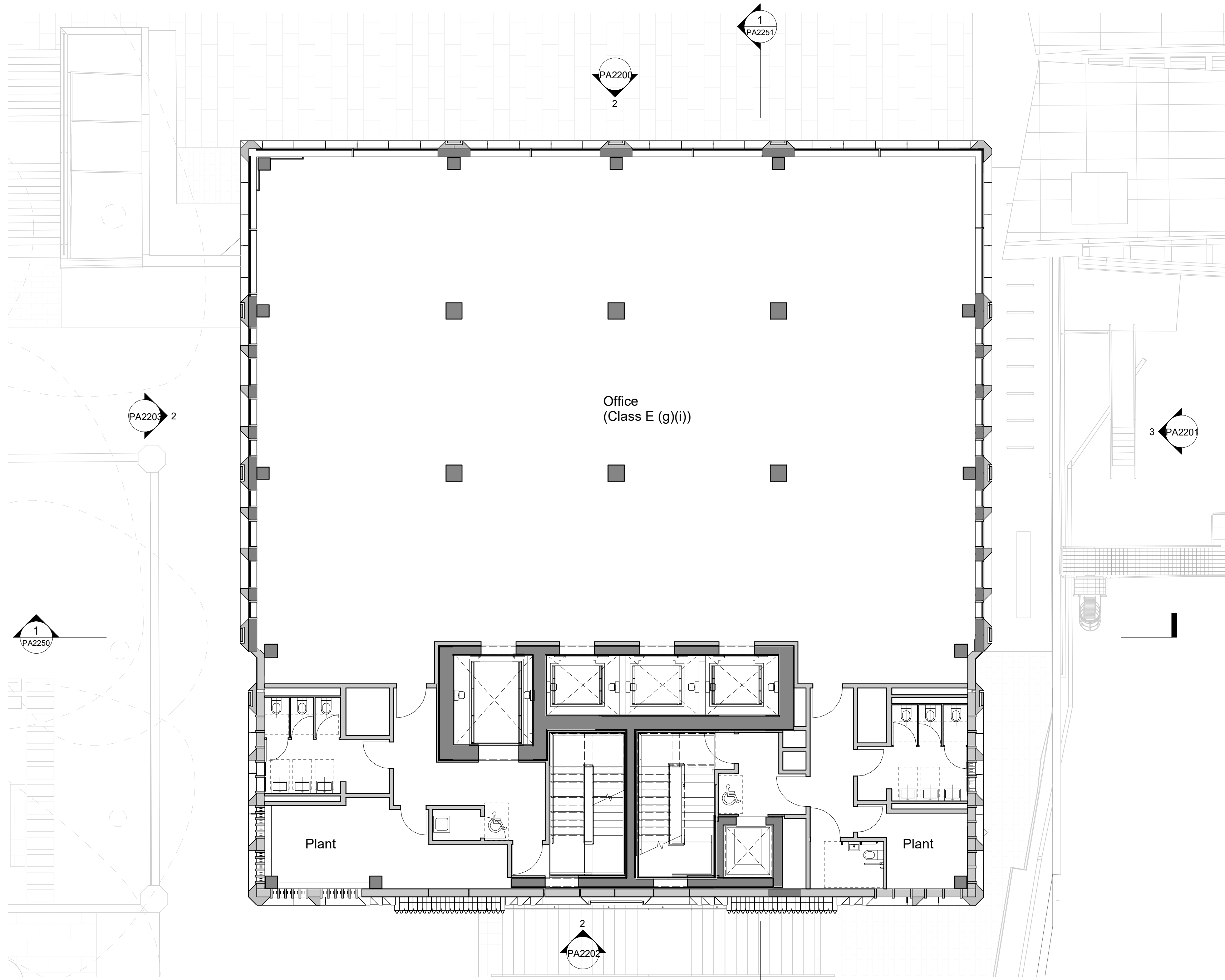
03 Level 16 1 : 100
