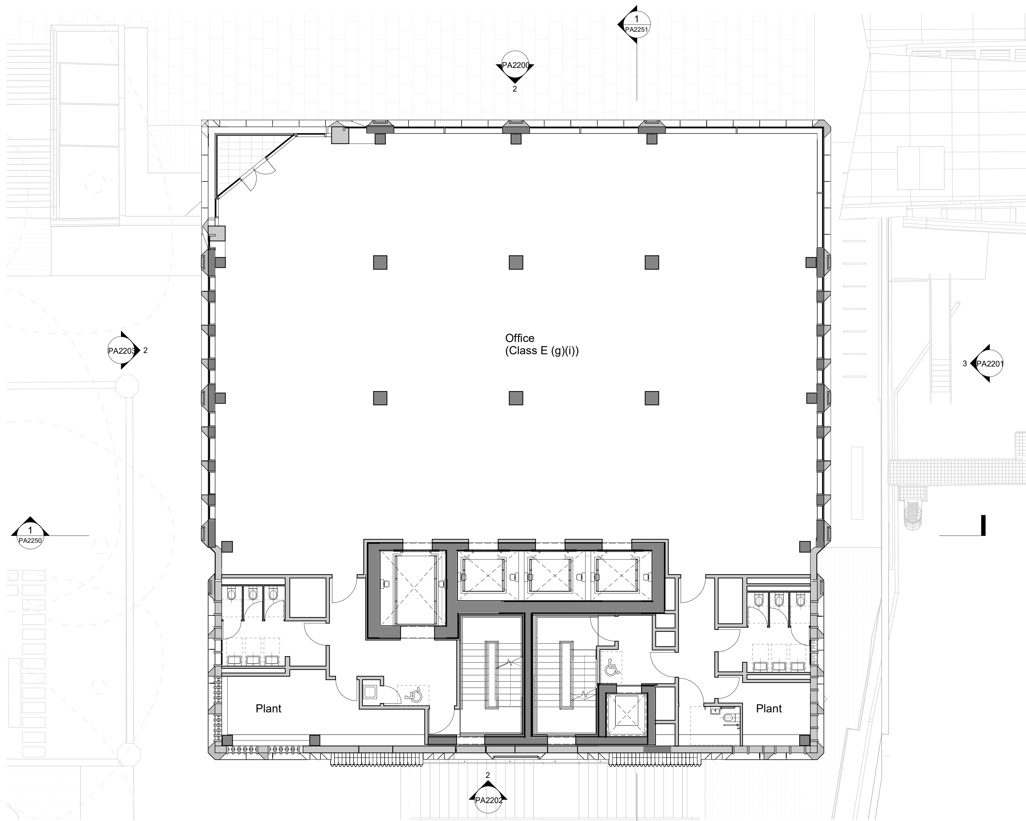
01 Level 14 1 : 100
