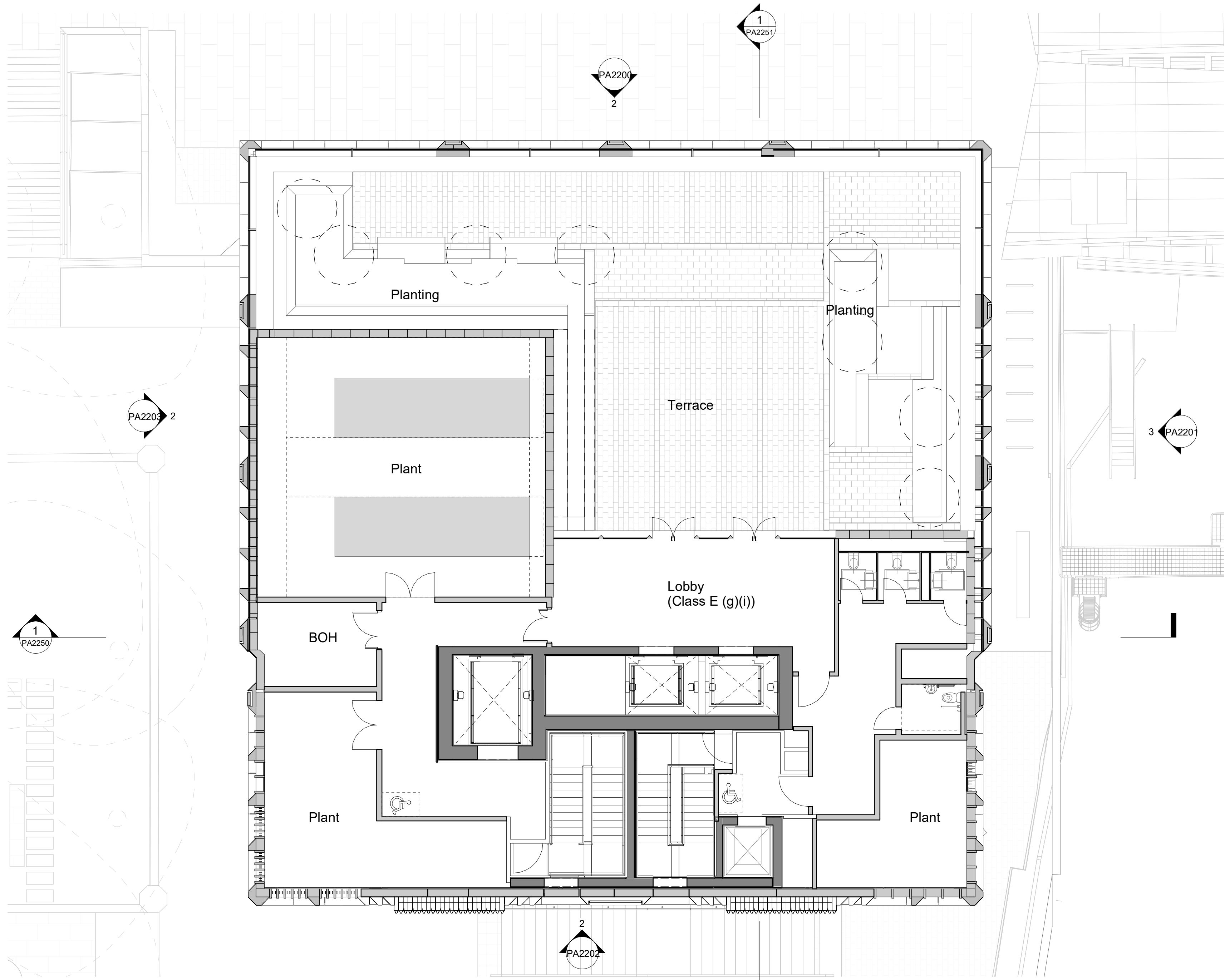
04 Level 17 1 : 100
