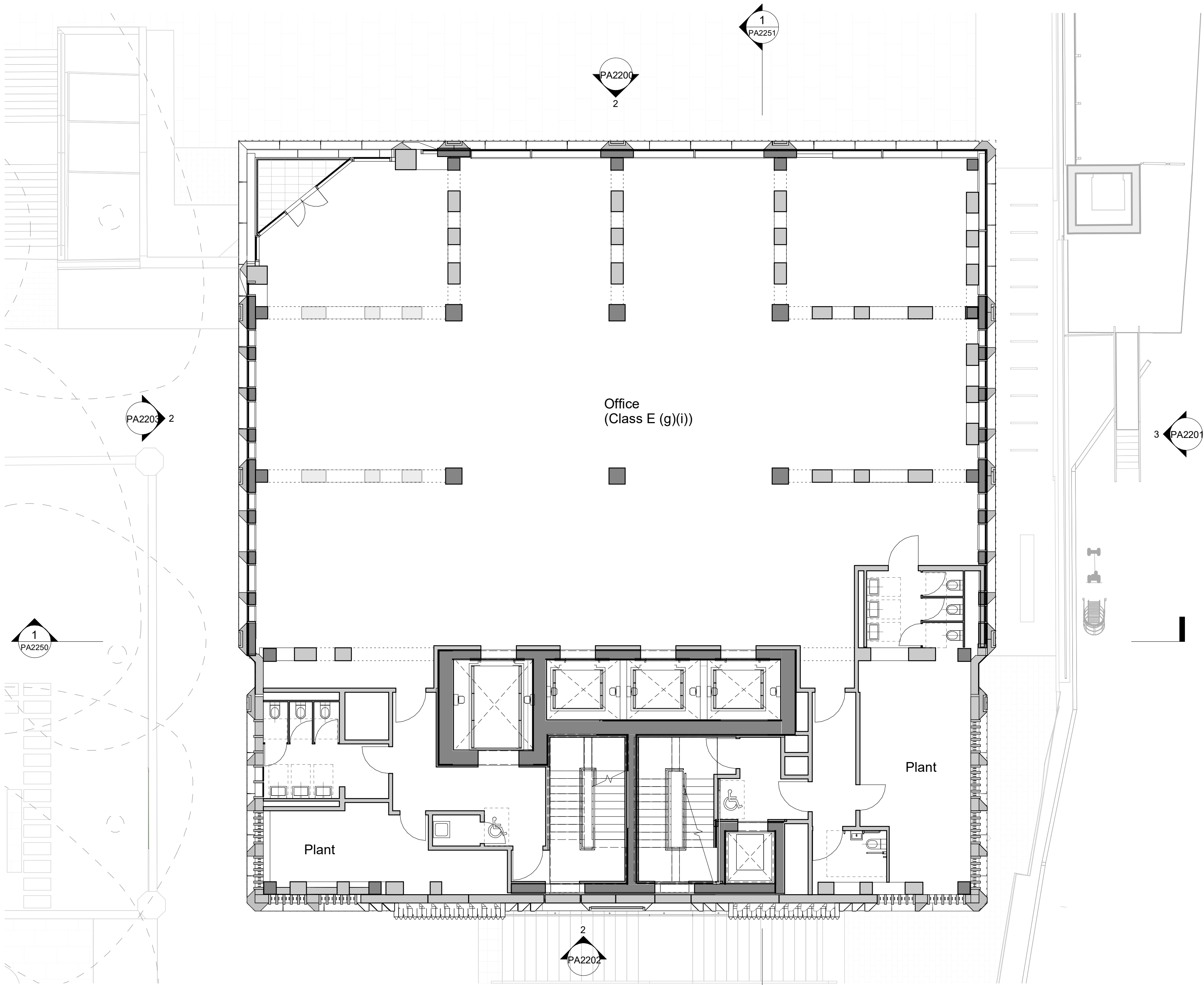
01 Level 02 1 : 100
