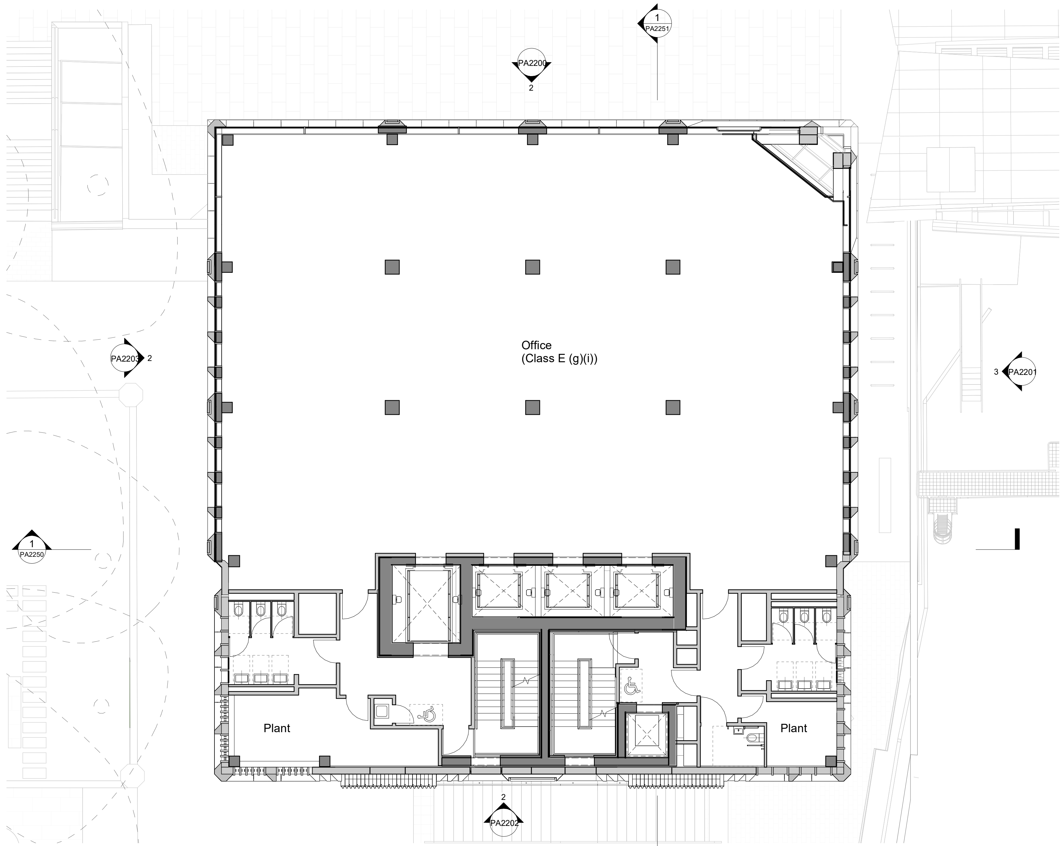
04 Level 05 1 : 100
