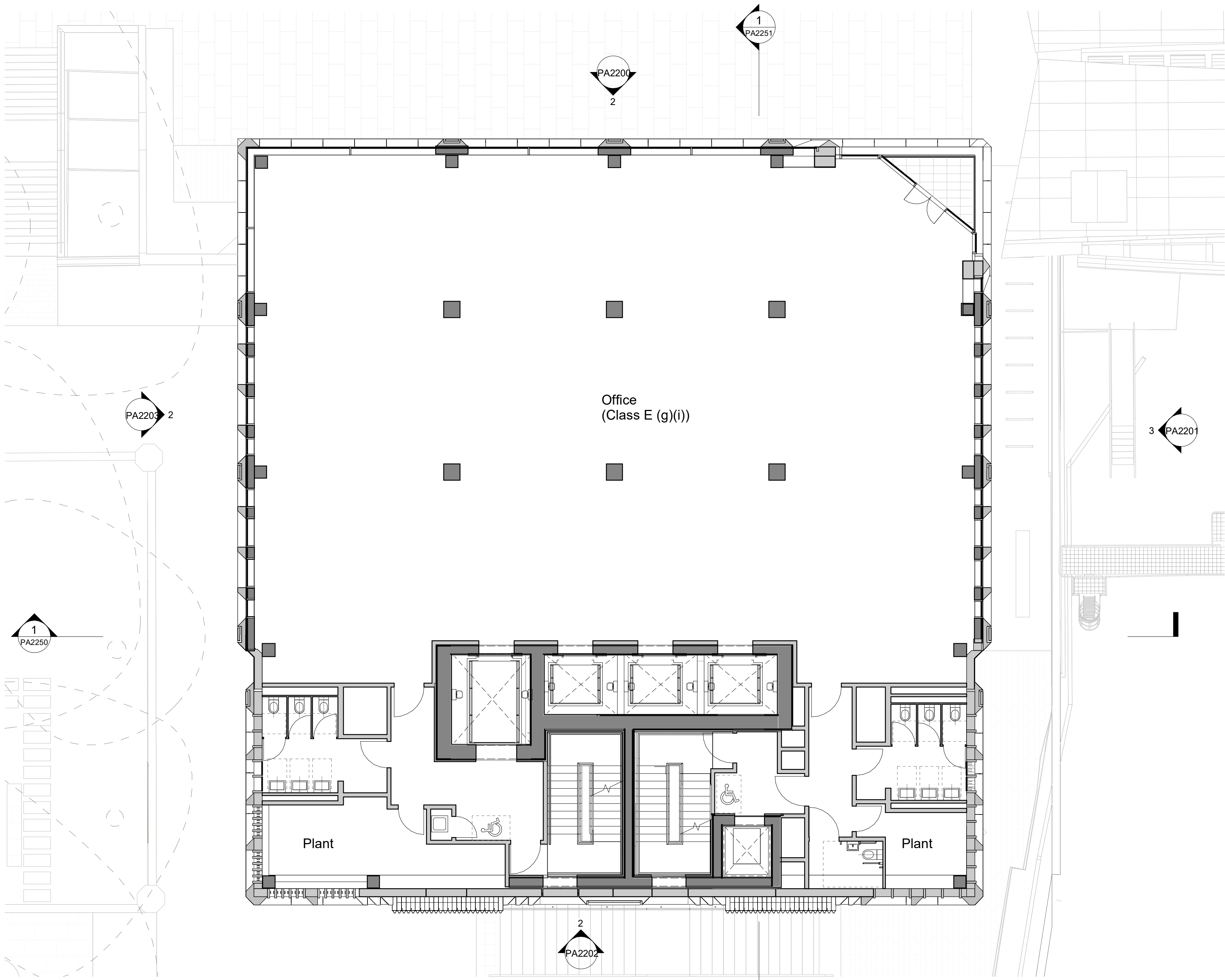
03 Level 04 1 : 100
