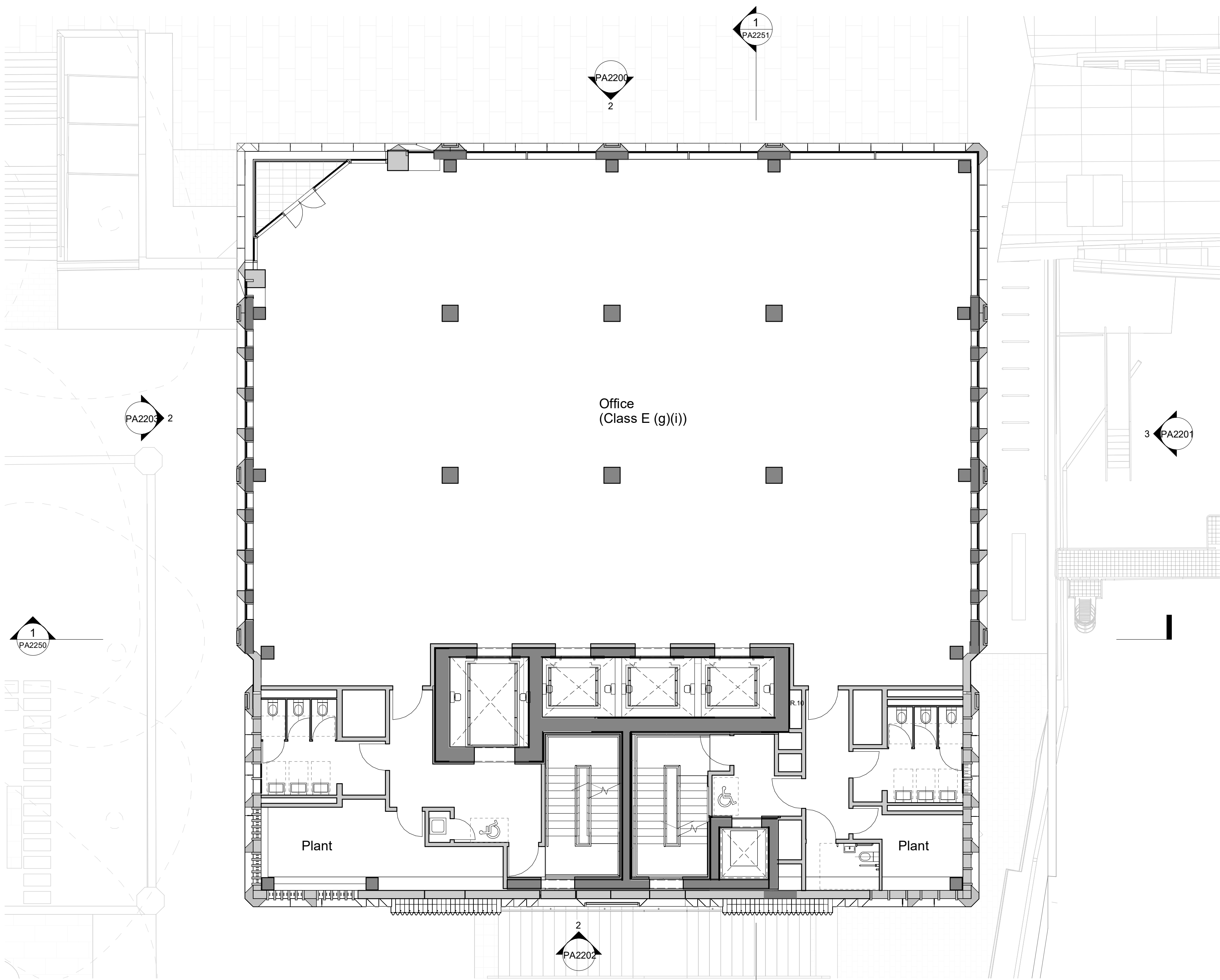
01 Level 10 1 : 100
