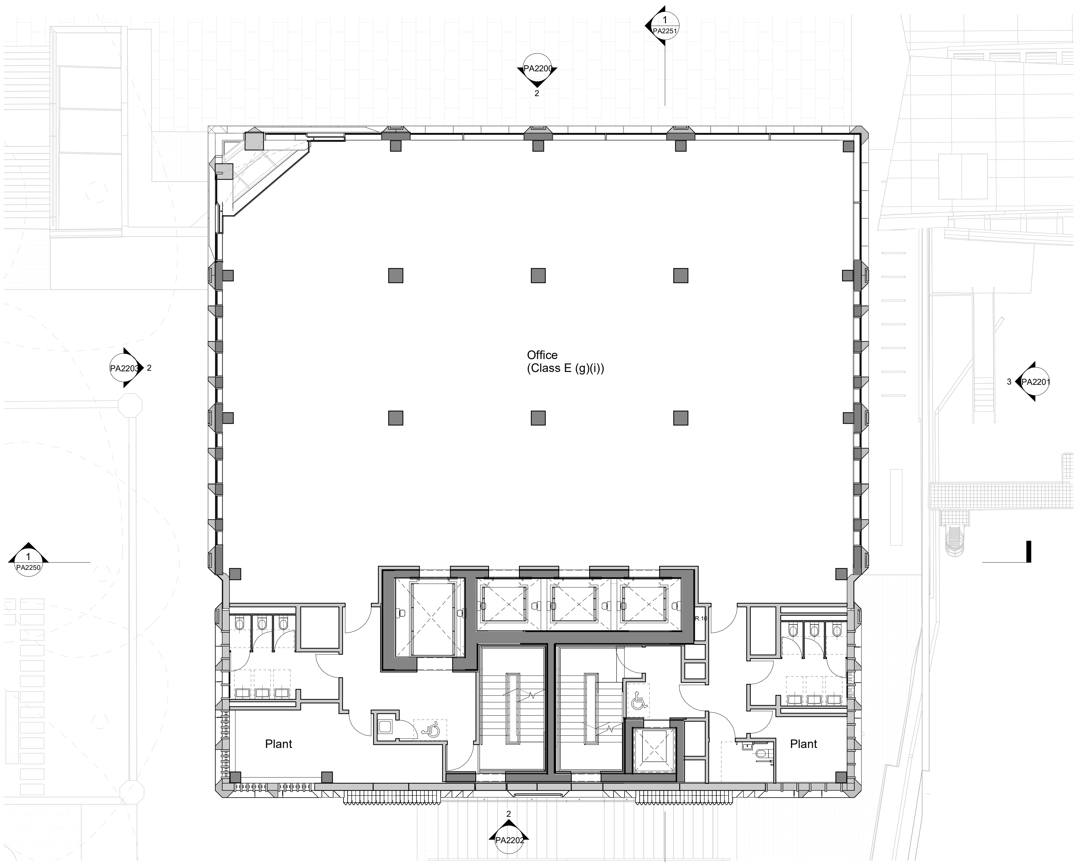
02 Level 11 1 : 100
