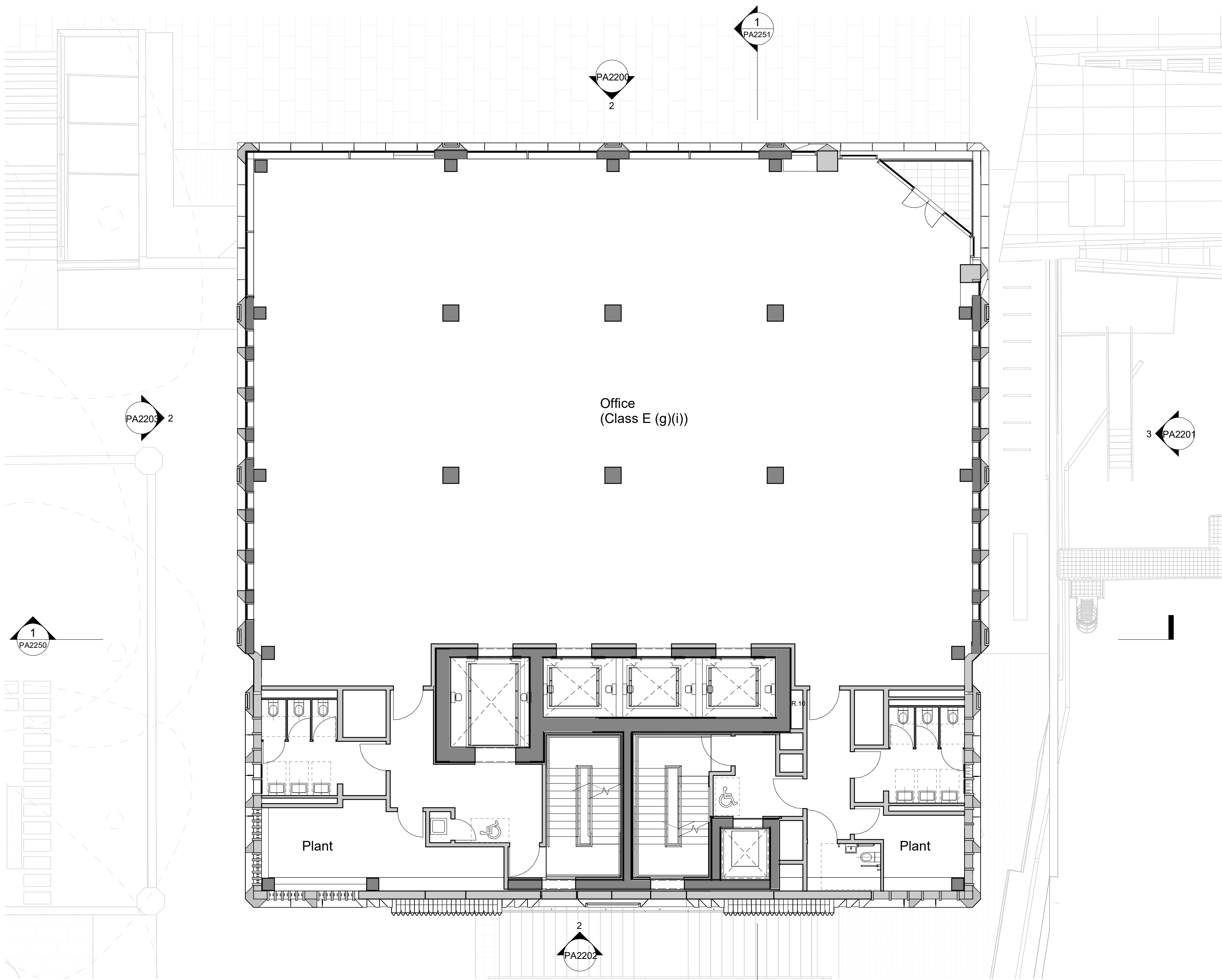
03 Level 12 1 : 100
