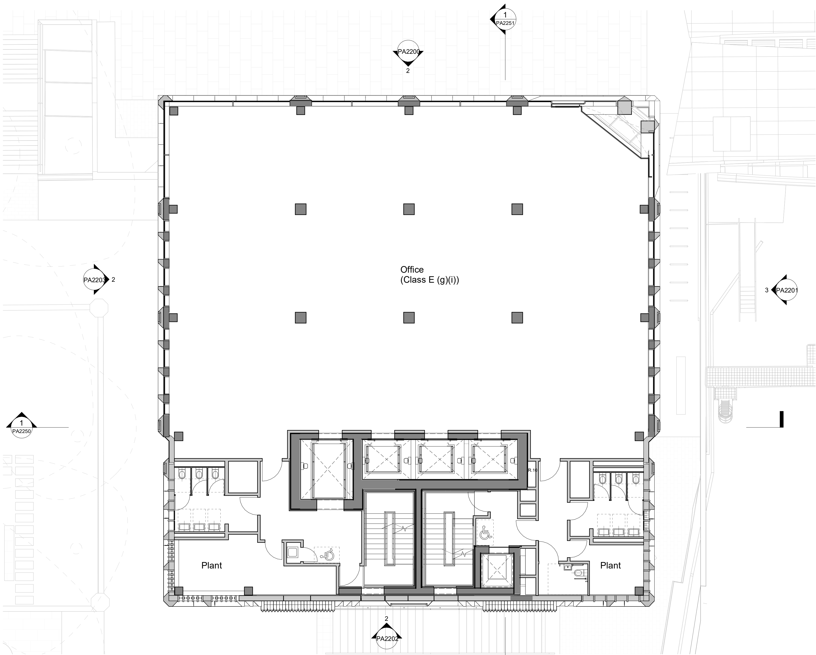
04 Level 13 1 : 100
