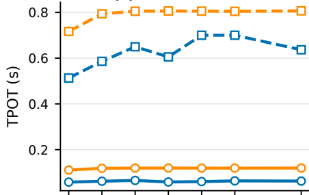
(f) LLaMA-13B TPOT
