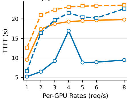
(e) LLaMA-13B TTFT
