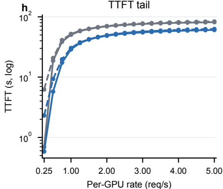
LLaMA2-13B + LongBench 4K TTFT tail
