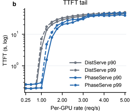
LLaMA2-13B + ShareGPT TTFT tail
