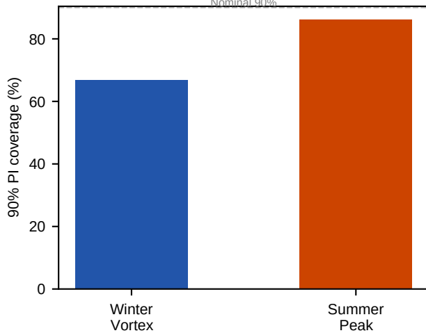
(d) Prediction interval coverage
