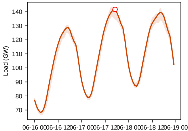
(d) Prediction interval coverage
