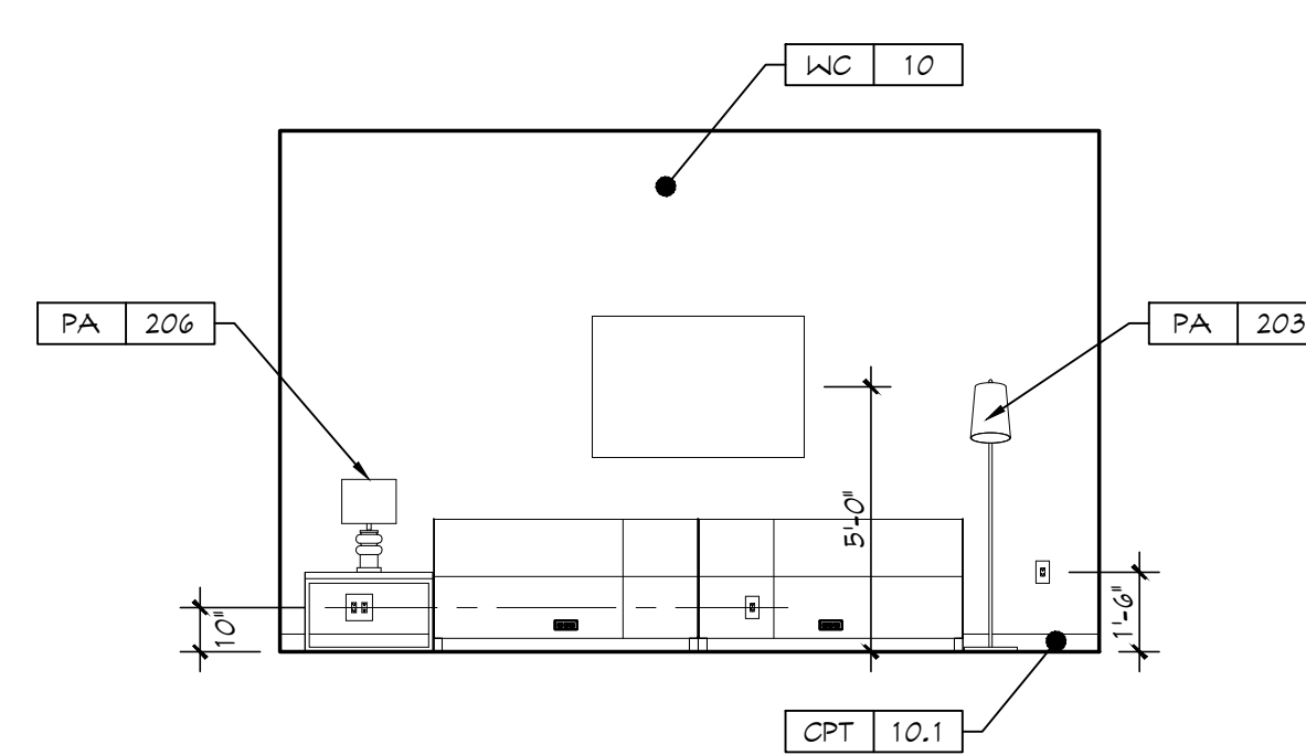
8 TV LOUNGE SCALE: 1/4" = 1'-0"
