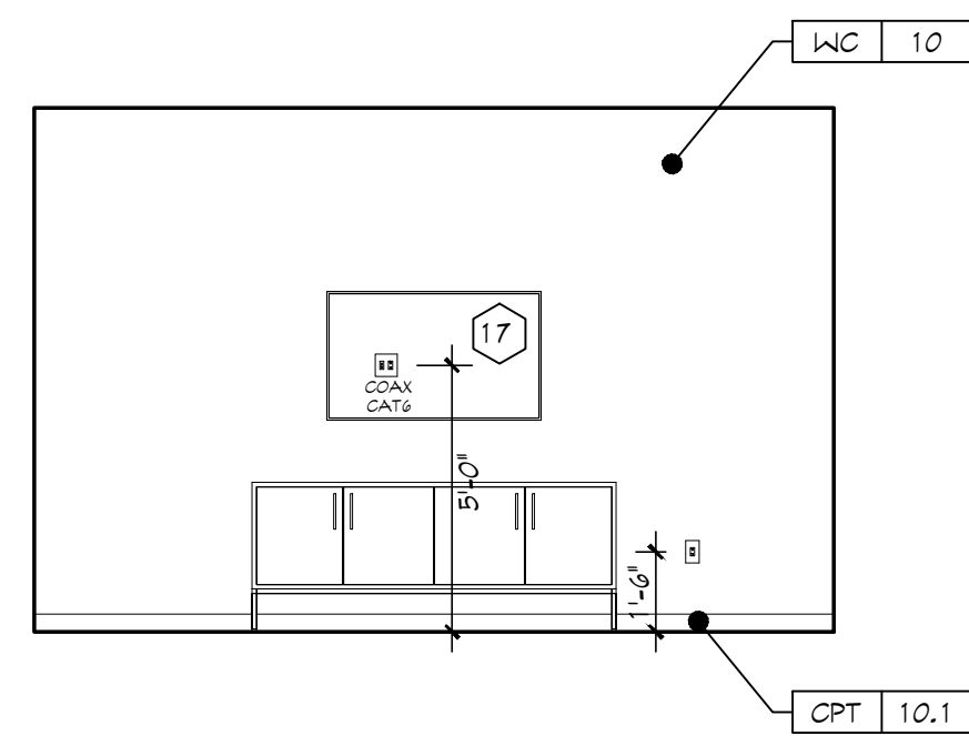
10 TV LOUNGE SCALE: 1/4" = 1'-0"
