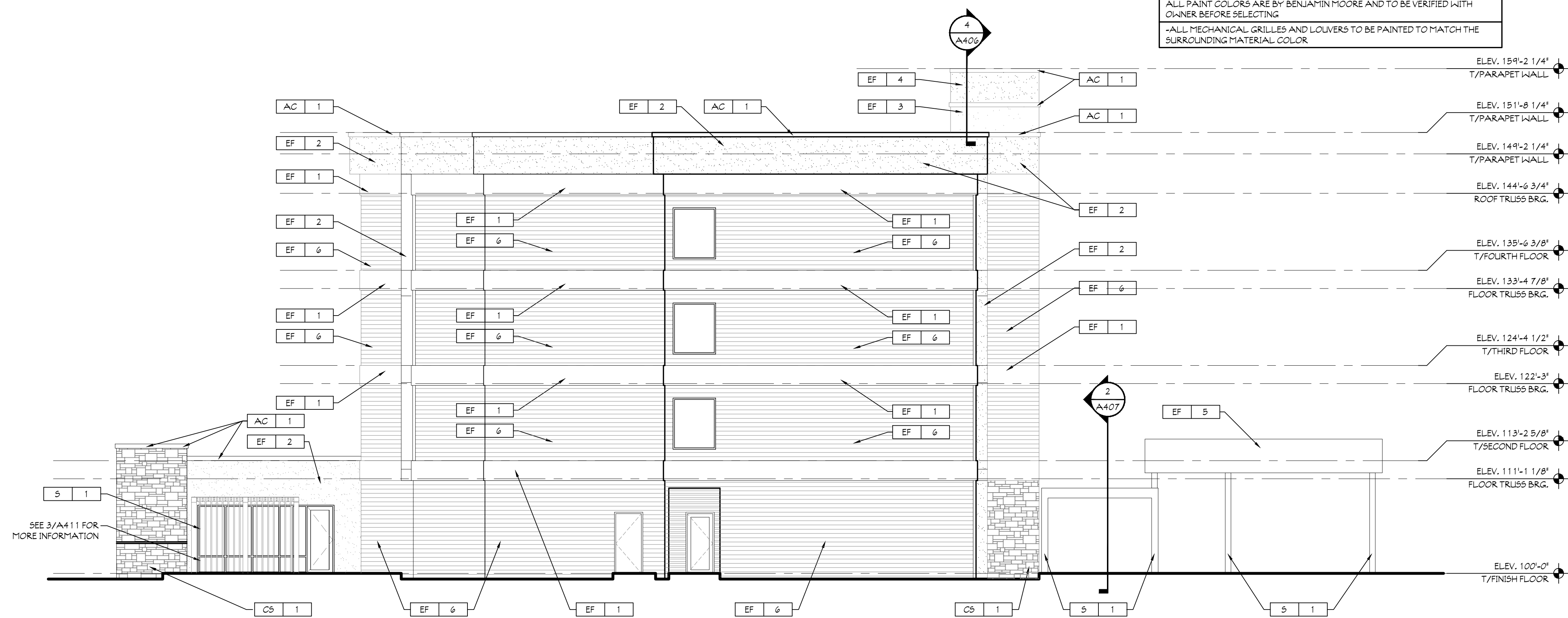
2 SIDE ELEVATION SCALE: 1/8" = 1'-0"
