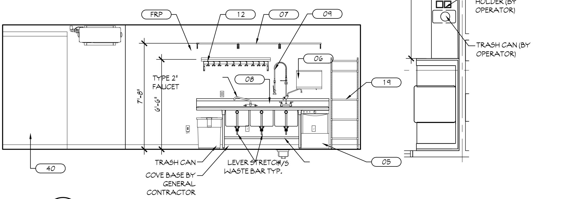
3 ELEVATION SCALE: 1/4" = 1'-0"
