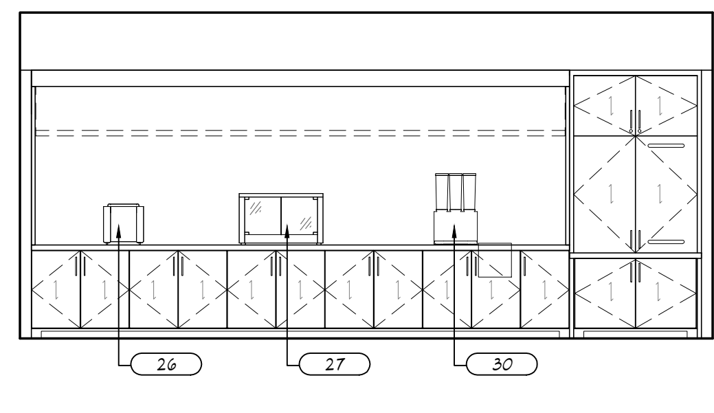
7 ELEVATION SCALE: 1/4" = 1'-0"
