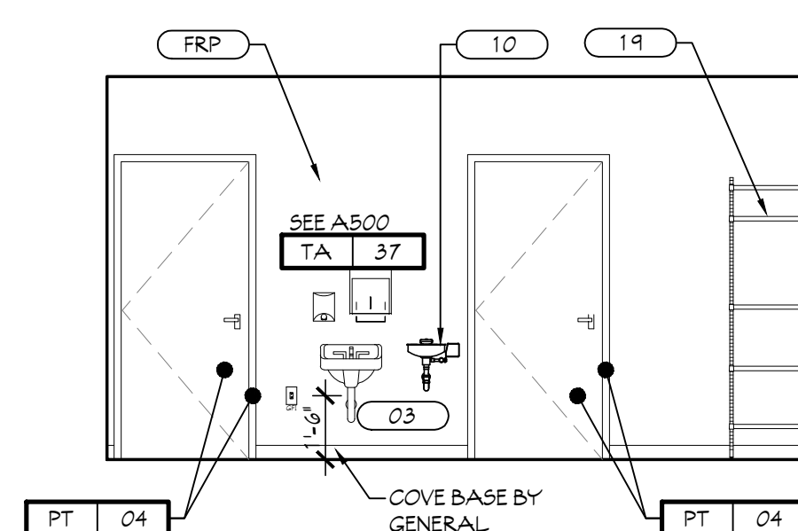
4 ELEVATION SCALE: 1/4" = 1'-0"
