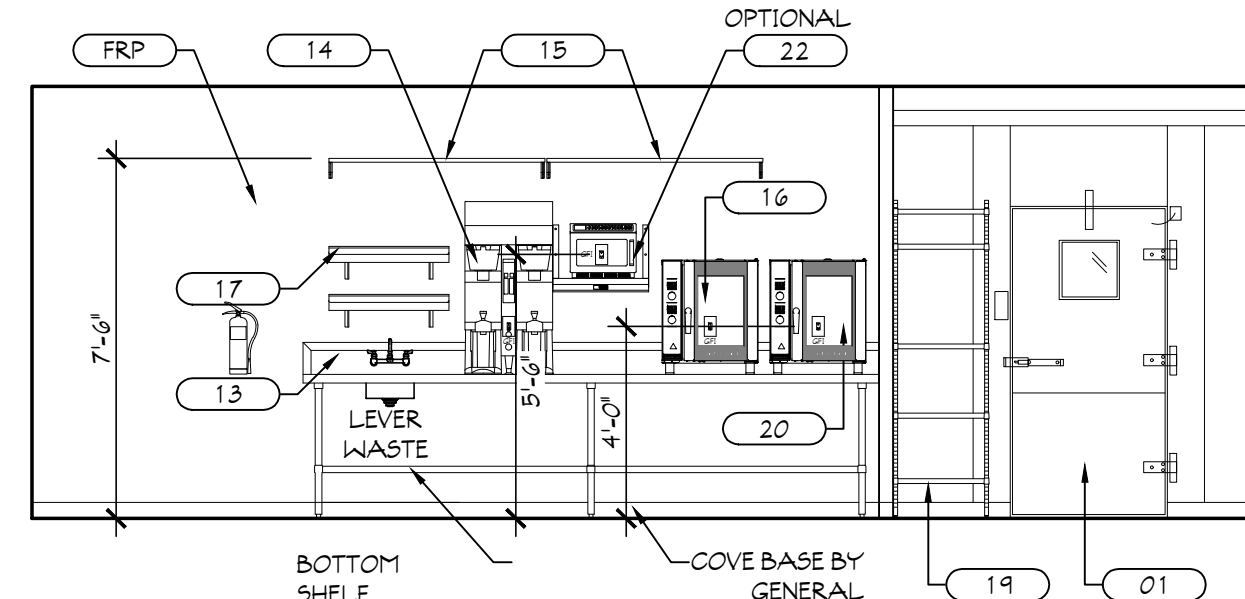
5 ELEVATION SCALE: 1/4" = 1'-0"
