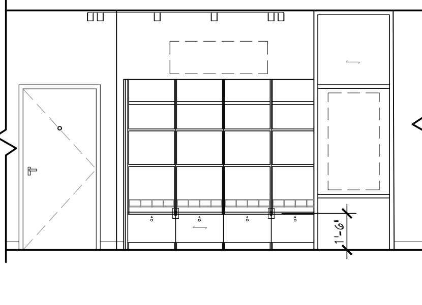
9 ELEVATION SCALE: 1/4" = 1'-0"
