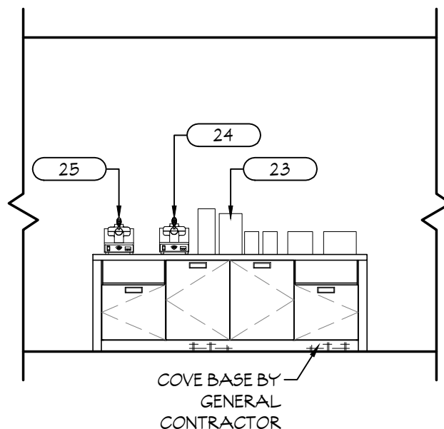
8 ELEVATION SCALE: 1/4" = 1'-0"
