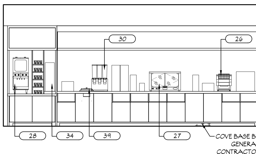
6 ELEVATION SCALE: 1/4" = 1'-0"
