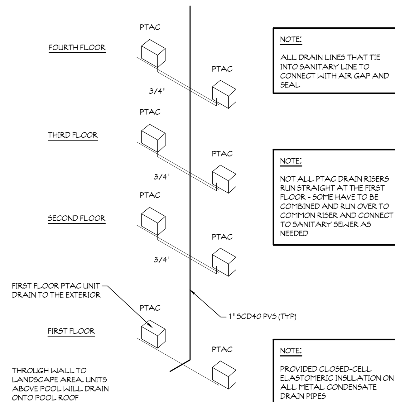
3 CONDENSATE DRAIN SCALE: NOT TO SCALE
