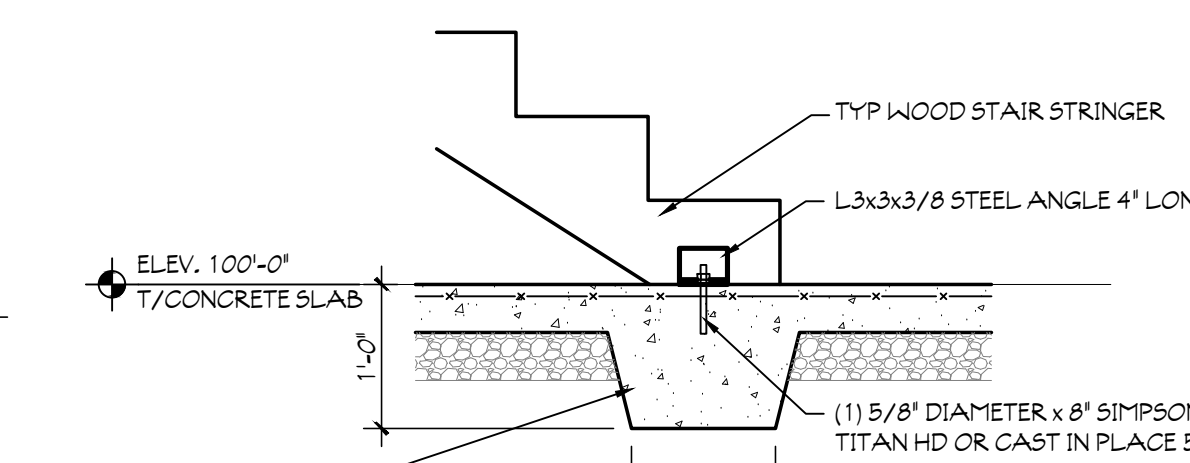
11 STAIR STRINGER SCALE: 3/4" = 1'-0"
