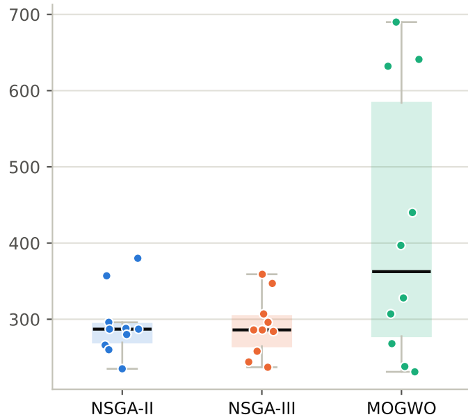
Najlepszy makespan [tiki]
