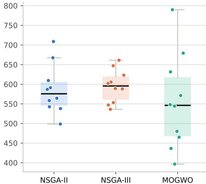
Najlepsza energia
