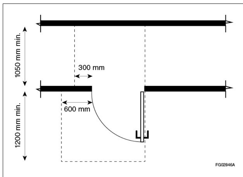
Figure A-3.8.4.3.-A
