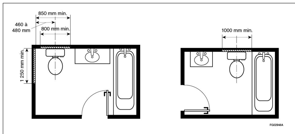
Figure A-3.8.4.5. 4)
