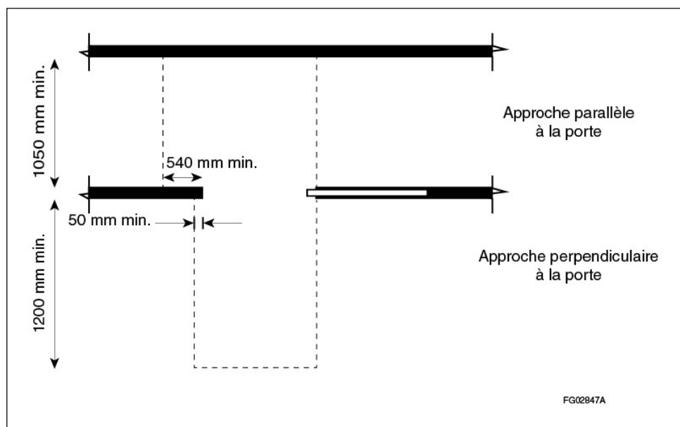
Figure A-3.8.4.3.-B
