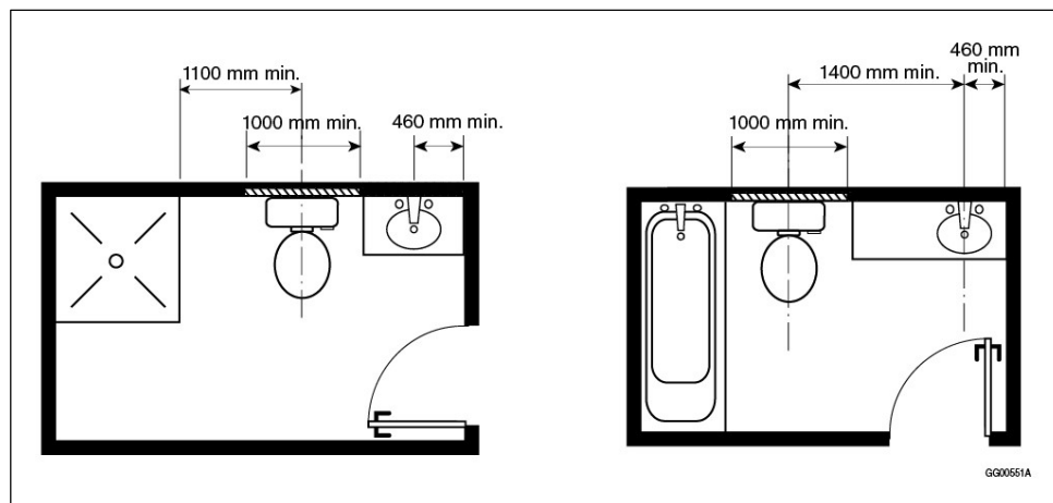
Figure A-3.8.5.5. 1)
