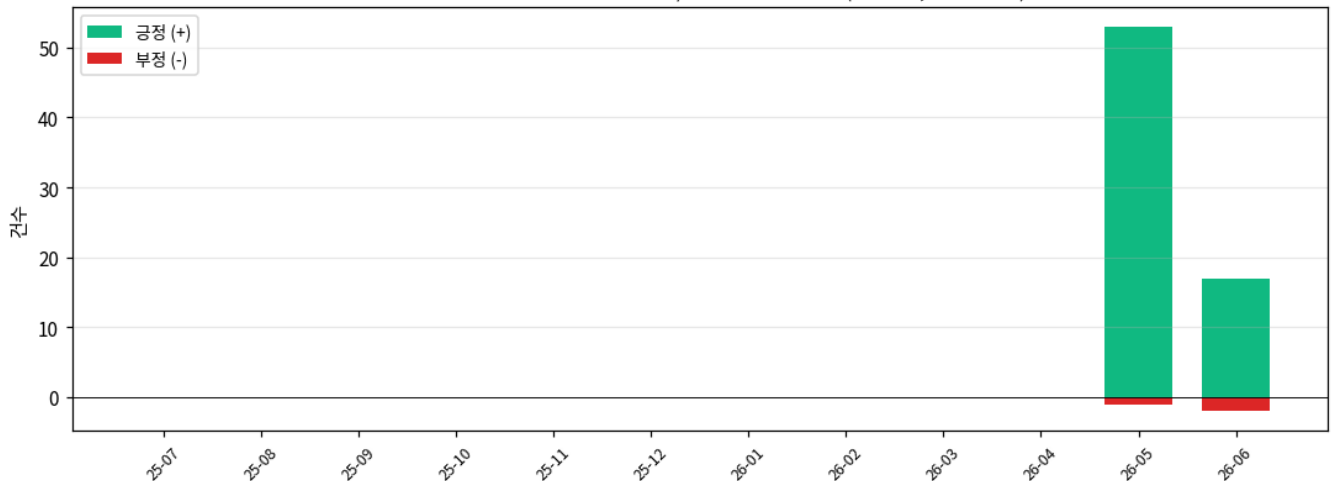
SNOW — 최근 12개월 월별 공시/뉴스 sentiment (긍정 위, 부정 아래)
