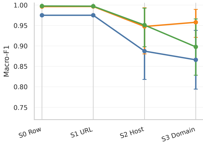
ISCX-URL2016
