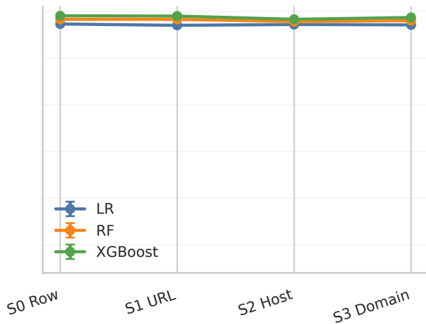
PhiUSIIL
