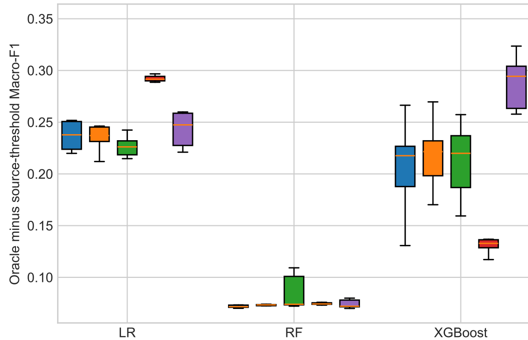
ISCX-URL2016 to PhiUSIIL
