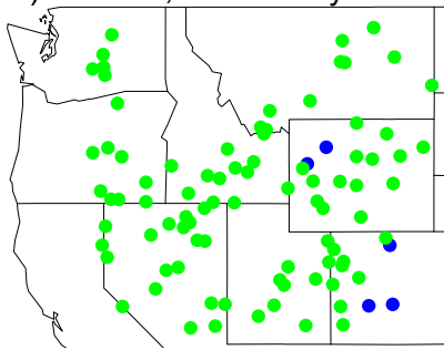
E) RCP8.5, endcentury
