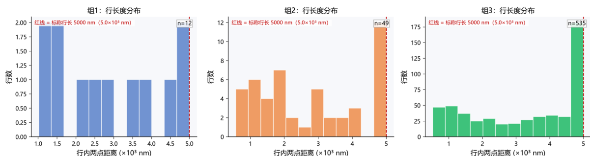
图 3: 三组行长度分布直方图（红色虚线为标称行长 5000nm）
