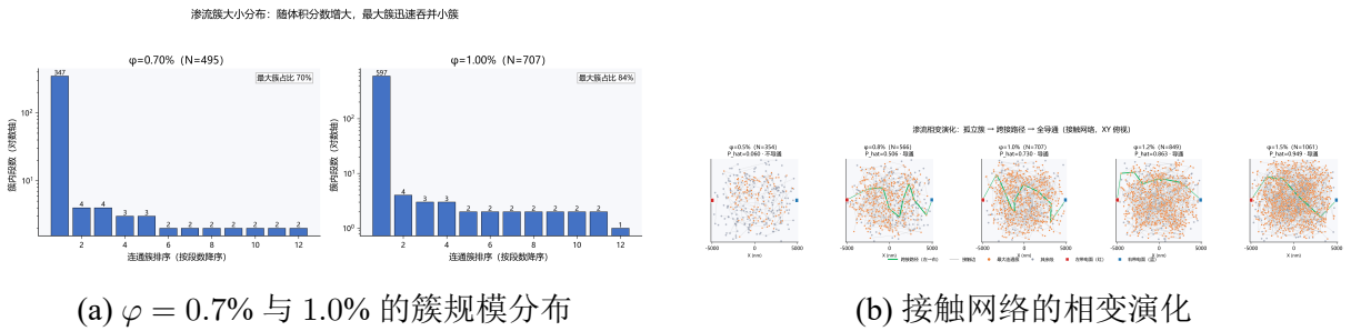
图 9: 渗流簇结构及相变演化特征
