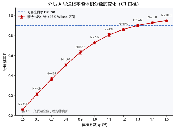
(a) P - \varphi 相变曲线
