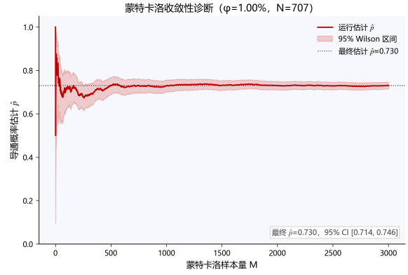
(b) \varphi = 1.00\% 处收敛曲线
