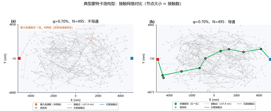
图 8: 典型导通与不导通构型的接触网络对比
