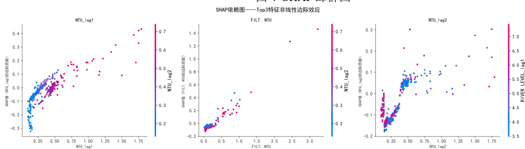
图5 SHAP 依赖图
