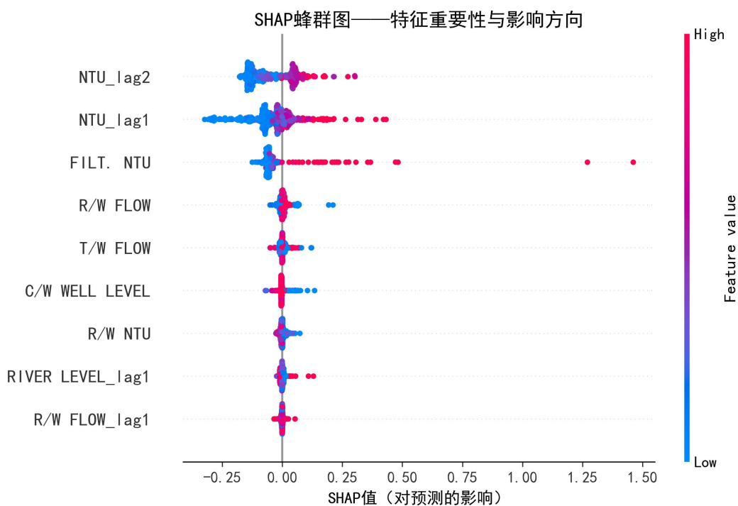
图4 SHAP 蜂群图
