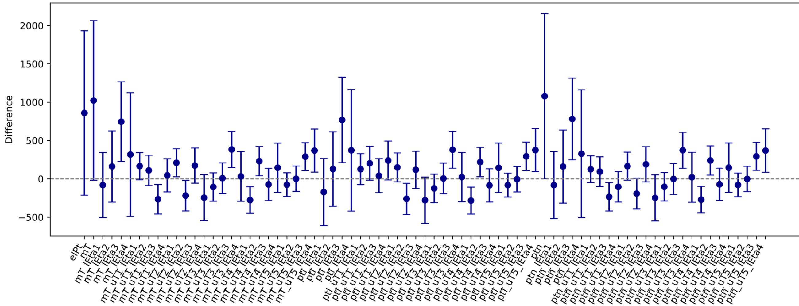
13 TeV: (W^+ \rightarrow e\nu) - (W^- \rightarrow e\nu)
