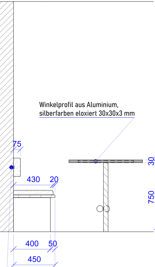
Schnitt C - C
