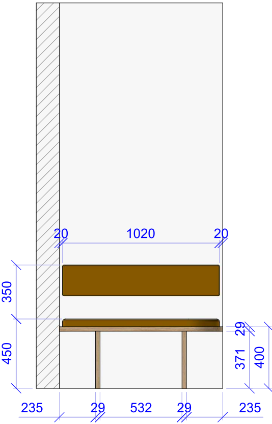
Schnitt B - B
