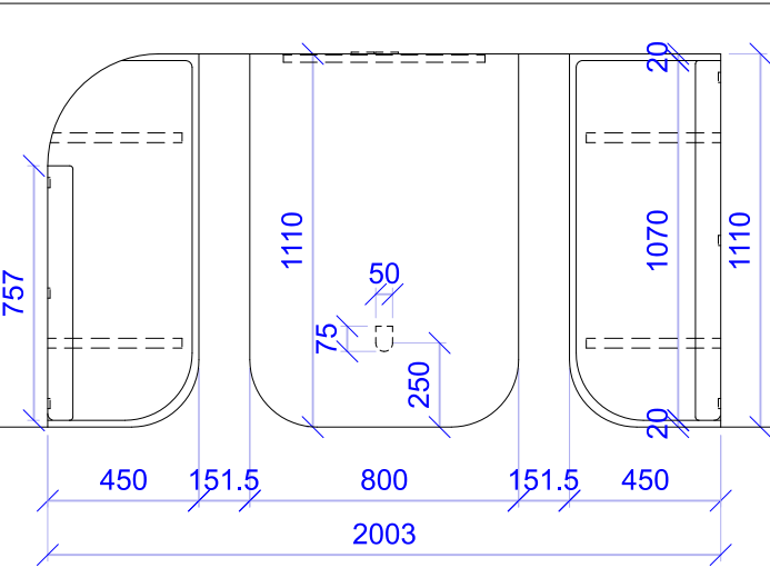
Draufsicht
