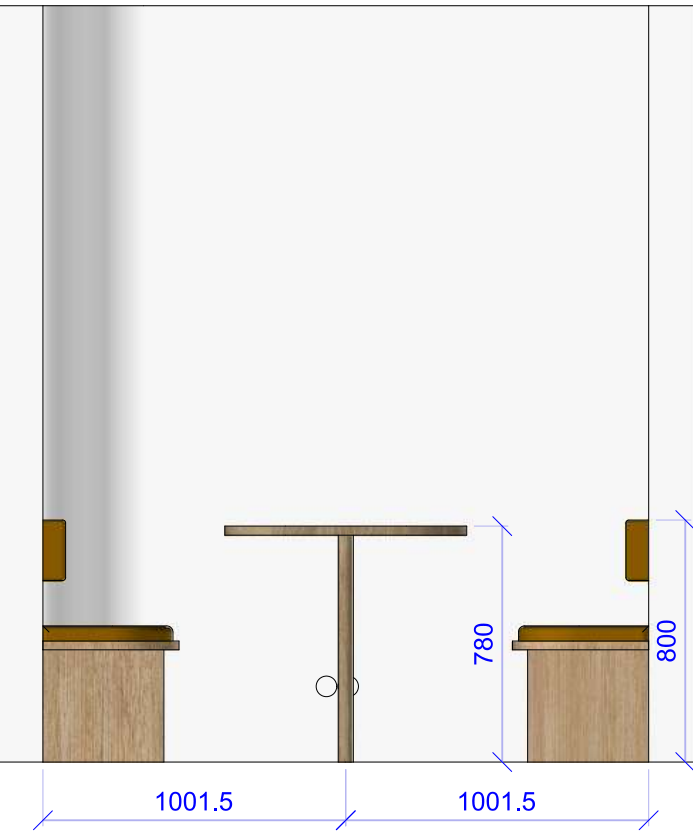
Vorderansicht
