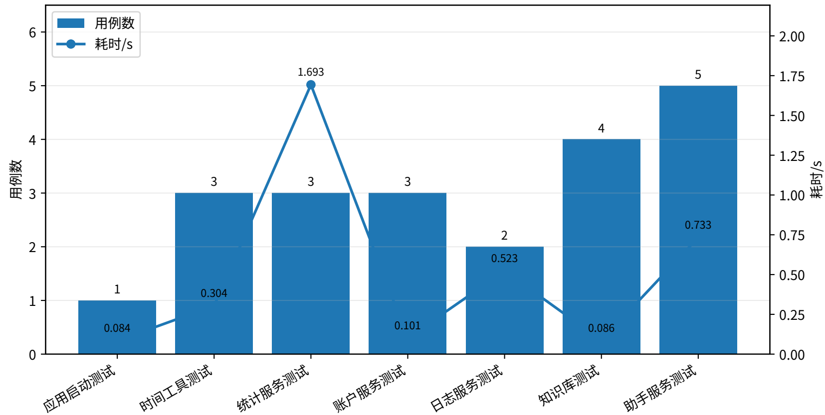
后端自动化测试用例数与耗时对比
