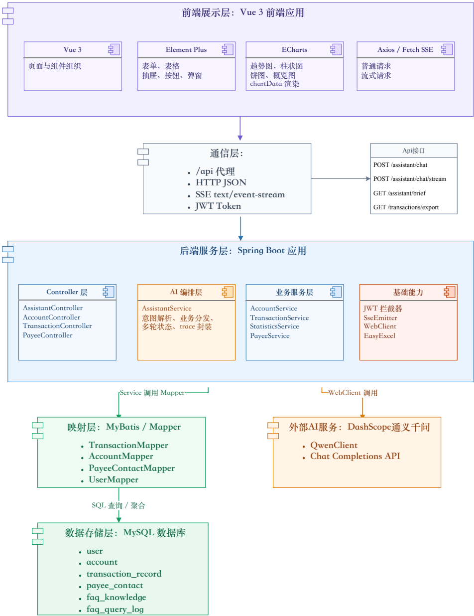
图 3.1 系统技术栈架构图
