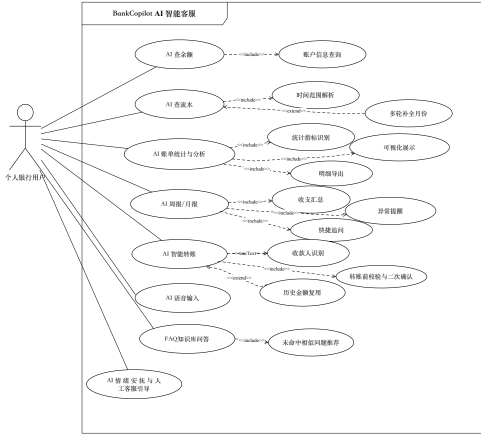
图 4.1 AI 智能客服用例图
