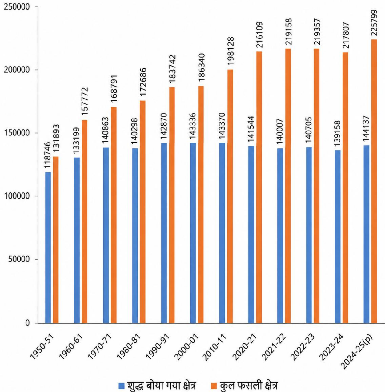
चित्र 15: शुद्ध बोया गया क्षेत्र, कुल फसली क्षेत्र की प्रवृत्ति (1950-51 से 2024-25 (p))
