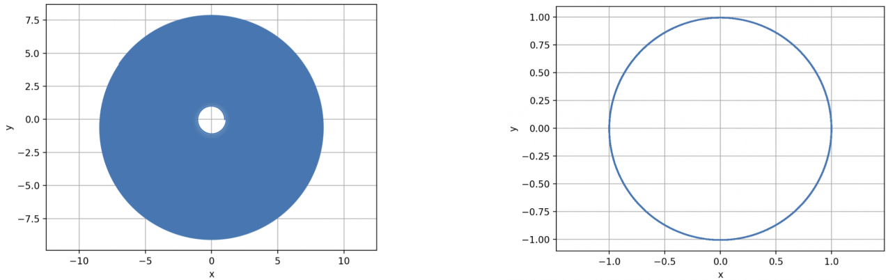
Figur 2: Explicit Euler (vänster) och semi-implicit Euler (höger), h = 0,01 , T = 10\,000 .
