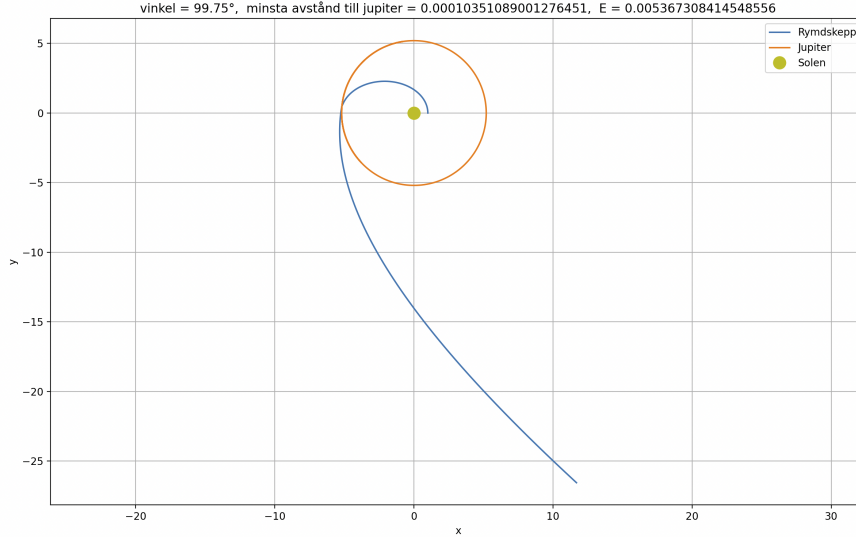
Figur 3: Skeppets bana med \theta = 99,75^\circ och h = 10^{-4} .
