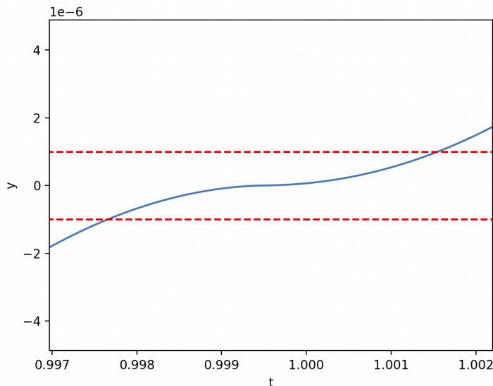
Figur 1: Numerisk lösning nära y = 0 . Streckade linjer: |y| = 10^{-6} .
