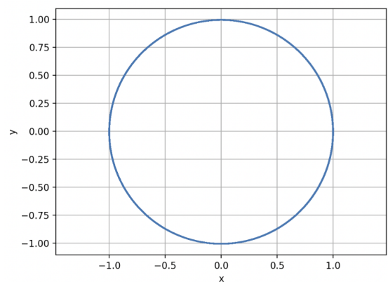
Figur 2: Explicit Euler (vänster) och semi-implicit Euler (höger), h = 0,01 , T = 10\,000 .
