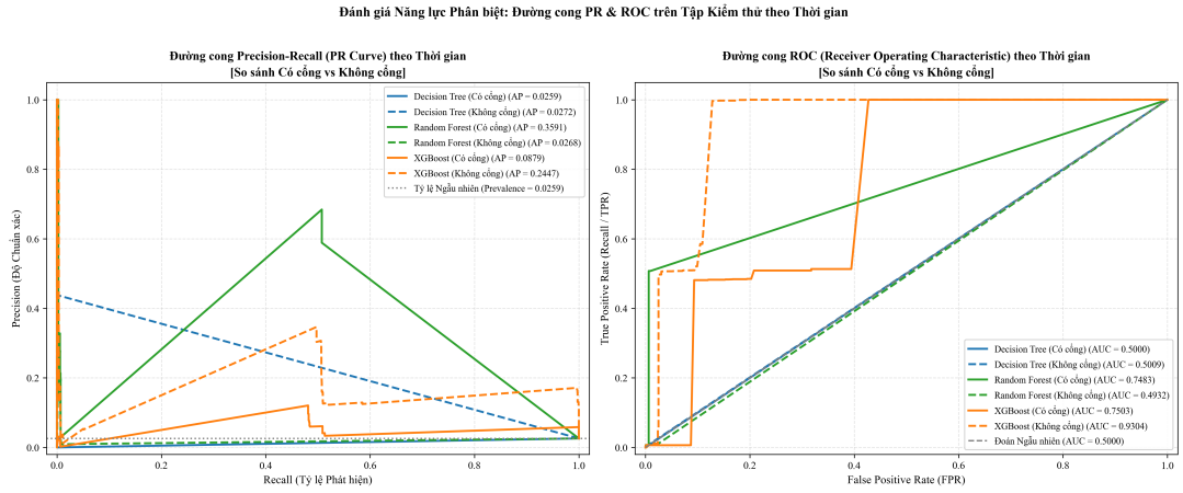
Hình 6.3: Đường cong ROC và Precision-Recall đối chiếu giữa các mô hình và kịch bản thực nghiệm, phản ánh sự biến thiên diện tích dưới đường cong khi có và không có đặc trưng công mạng.
