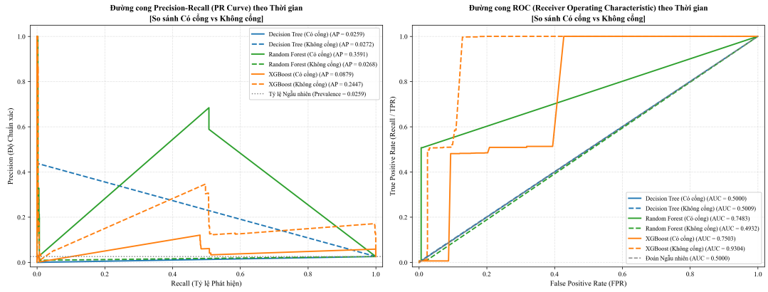
Hình 6.3: Đường cong ROC và Precision-Recall đối chiếu giữa các mô hình và kịch bản thực nghiệm, phản ánh sự biến thiên diện tích dưới đường cong khi có và không có đặc trưng công mạng.
