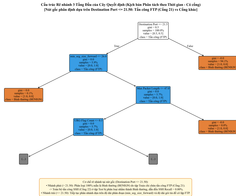
Hình 6.5: Cấu trúc 3 tầng đầu tiên của Decision Tree minh họa ngưỡng rẽ nhánh ưu tiên tại Destination Port \leq 21.5 .
