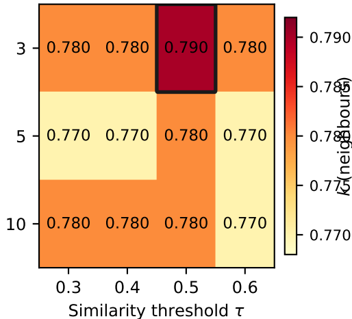
Macro F1 over HP grid (IHC, Full index)
