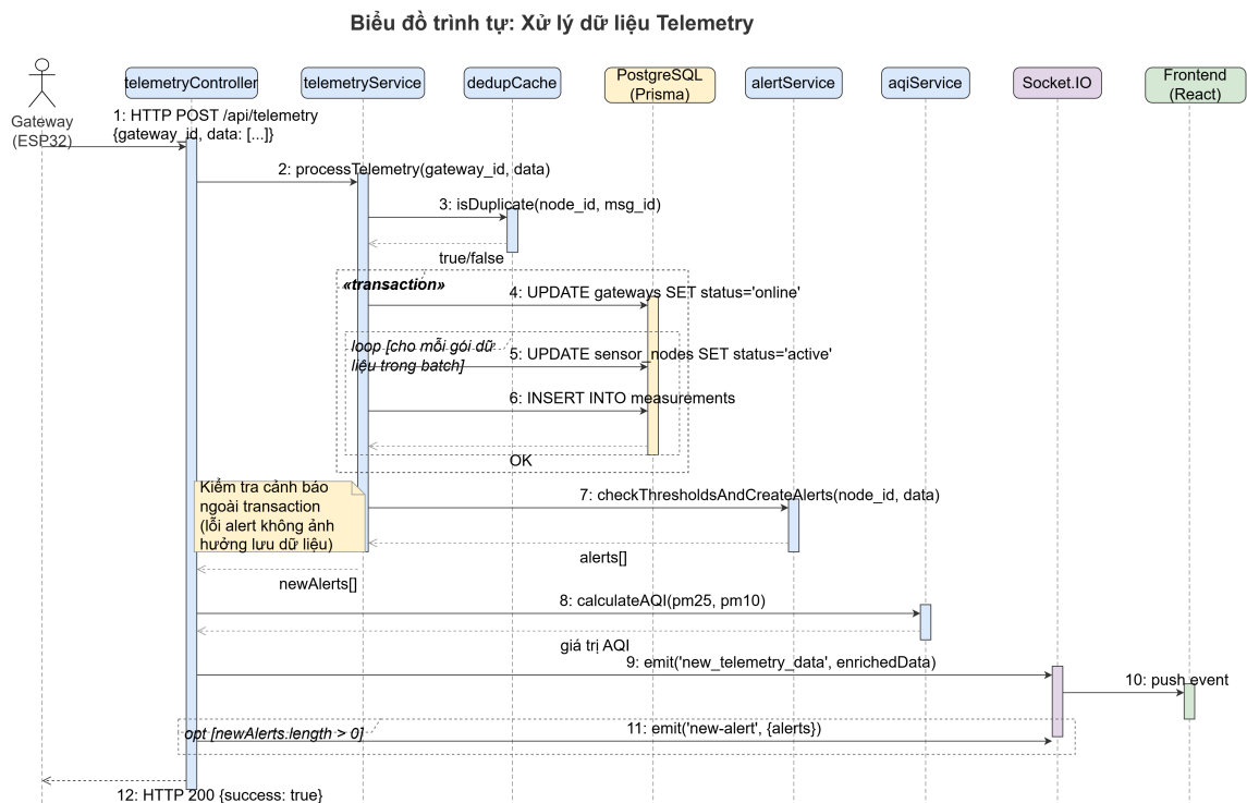
Hình 0.6: Biểu đồ trình tự xử lý dữ liệu Telemetry
