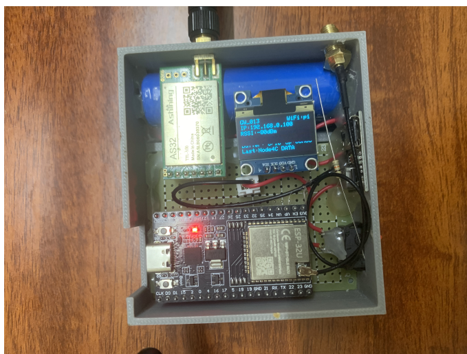
Hình 0.22: Gateway nhận gói tin từ Sensor Node 4C (NODE_076)
