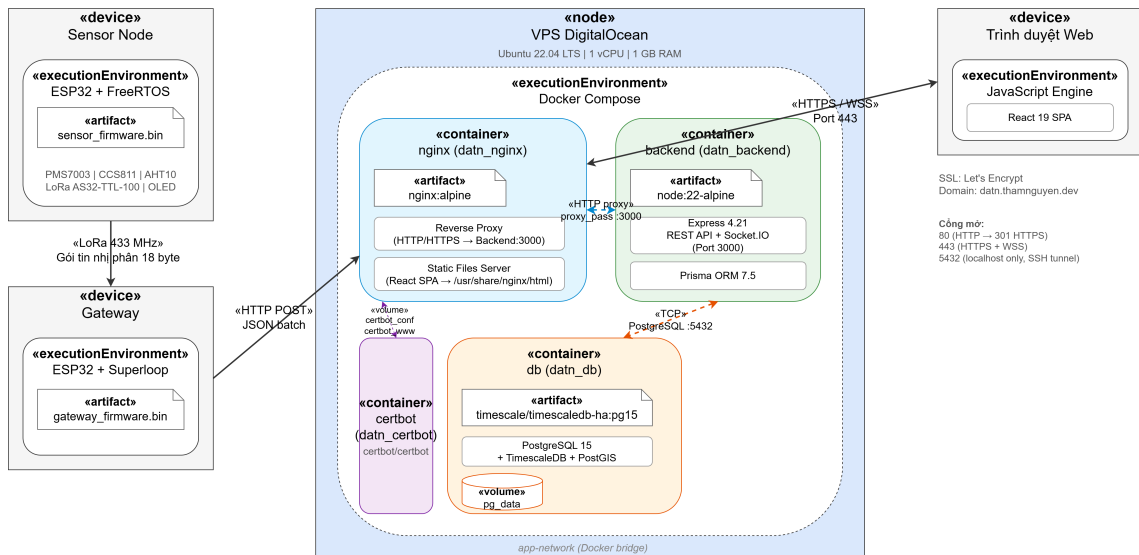
Hình 0.17: Biểu đồ triển khai hệ thống
