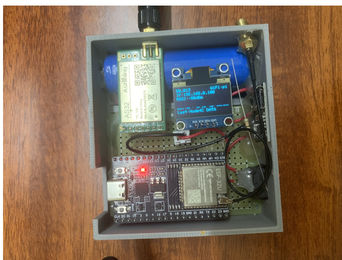
Hình 0.22: Gateway nhận gói tin từ Sensor Node 4C (NODE_076)
